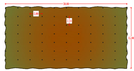
Plan 1:100
